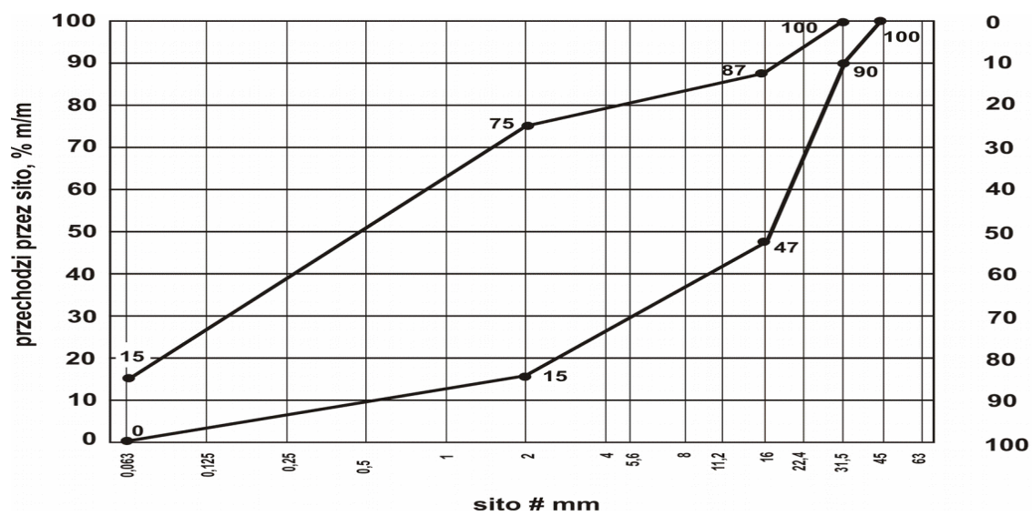
Rys. 4. Uziarnienie mieszanki niezwiązanej 0/31,5 dla nawierzchni
