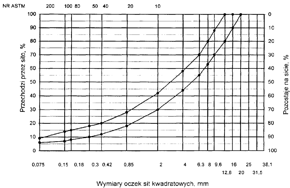
graniczne uziarnienia mieszanki mineralnej BA od 0 do 20 mm (mieszanka o nieciągłym uziarnieniu) do warstwy ścieralnej nawierzchni drogi o obciążeniu ruchem od KR3 do KR6 Rys. 6. Krzywe graniczne uziarnienia mieszanki mineralnej BA od 0 do 16 mm do warstwy ścieralnej nawierzchni drogi o obciążeniu ruchem od KR3 do KR6
